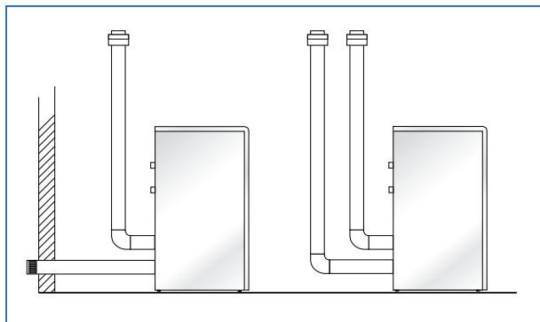
Rookgasafvoermogelijkheden
